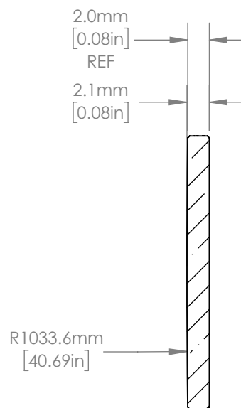
SECTION A-A SCALE 2 : 1
