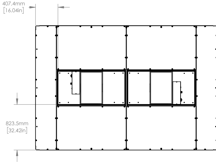
DIMENSIONS OF FAN UNIT
