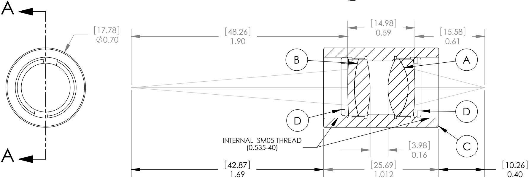
SECTION A-A
