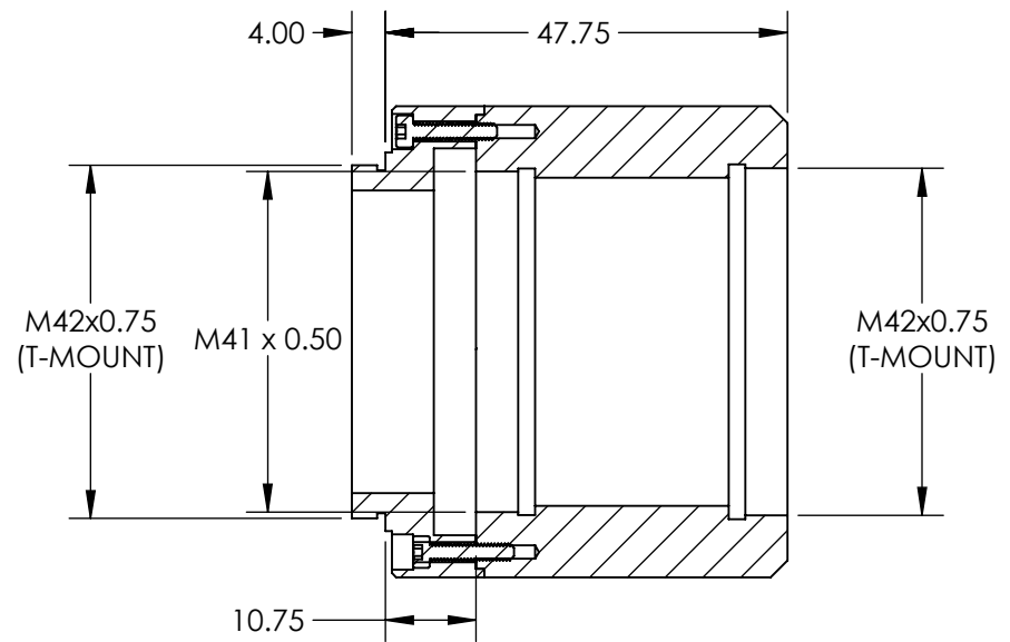
SECTION A-A
