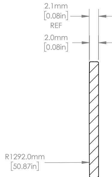
SECTION A-A SCALE 2 : 1
