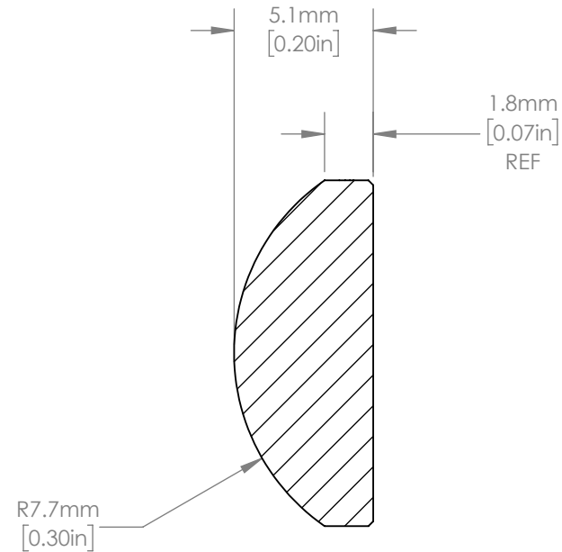
SECTION A-A SCALE 4 : 1
