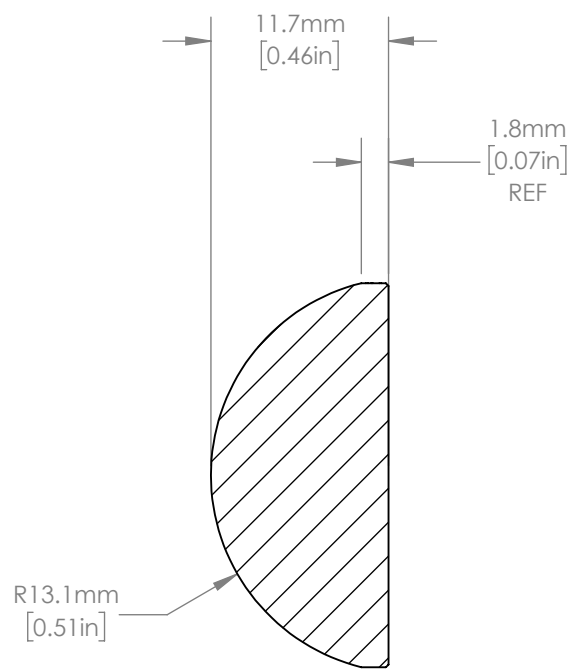
SECTION A-A SCALE 2 : 1
