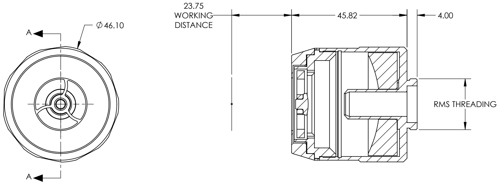
SECTION A-A
